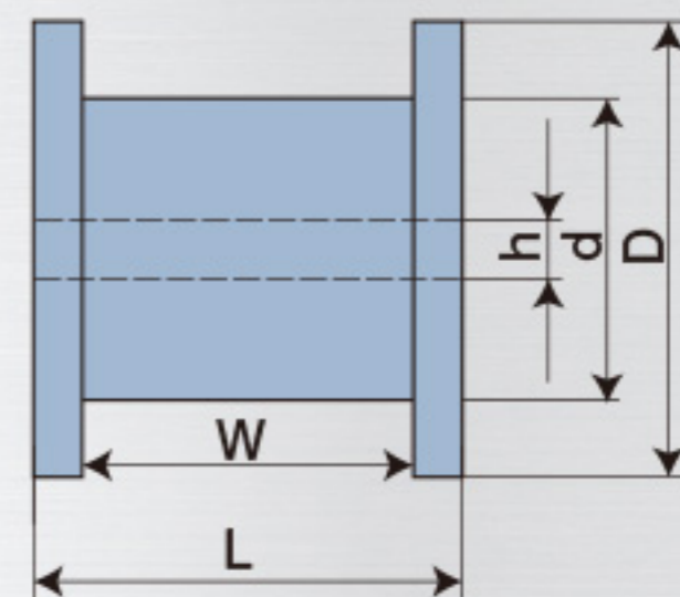
ボビン形状
